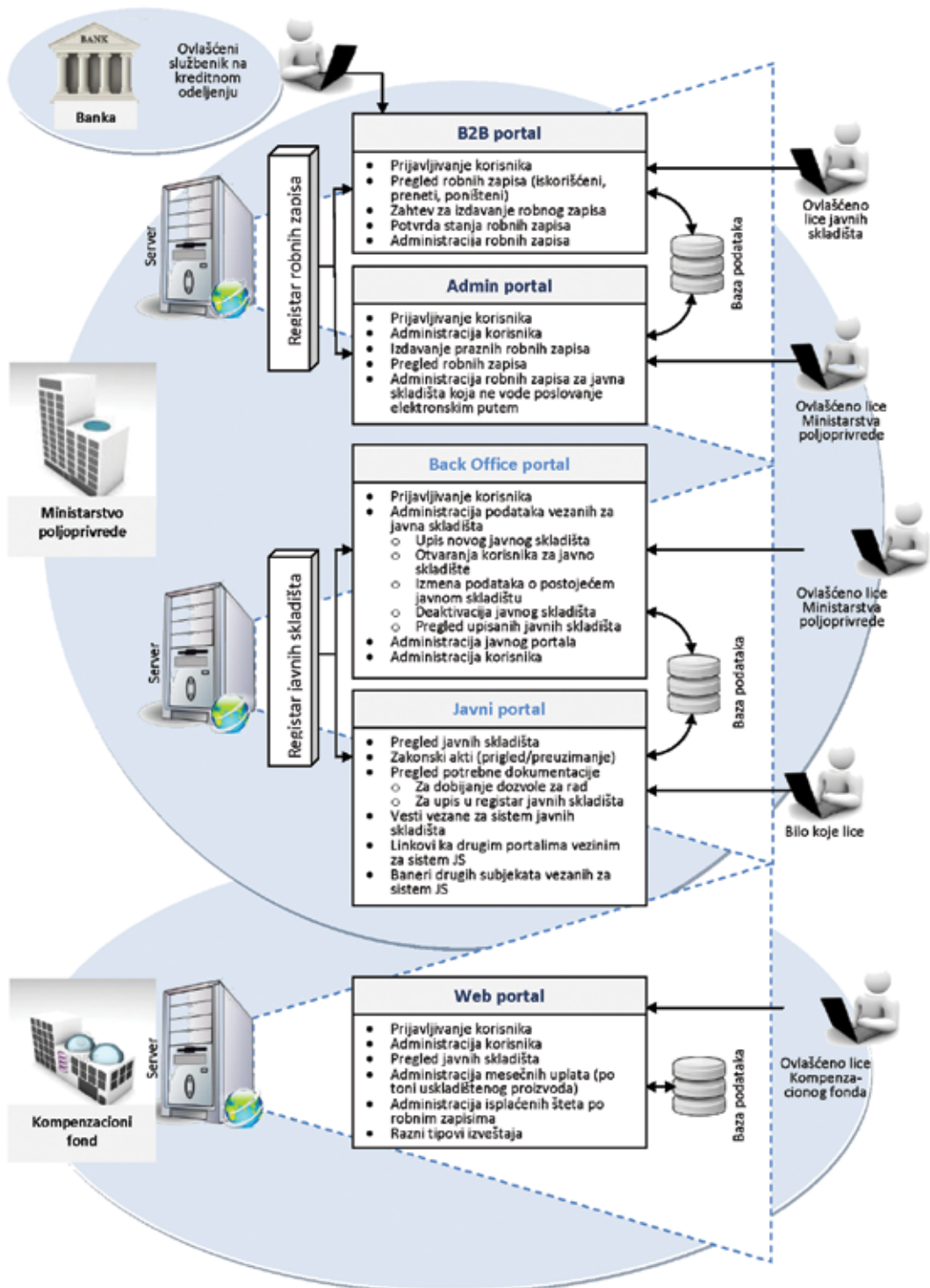
Slika 3.33 Informacioni sistem sistema javnih skladišta u Srbiji
