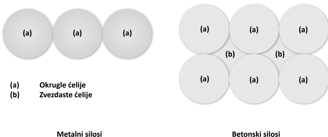
Slika 4.9 Uobičajeni oblici silosnih ćelija
