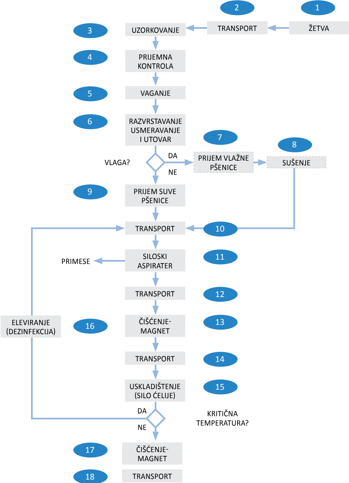
Slika 5.5 primer dijagrama toka procesa u skladištu za zrnaste kulture
