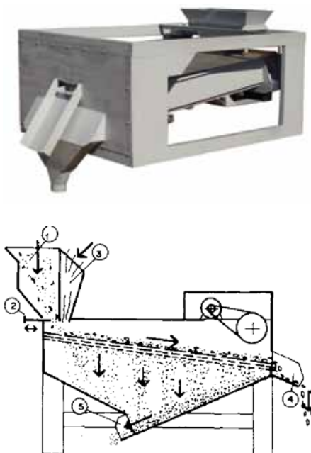
Slika 3.13 Izgled i šema silosnog aspiratera
