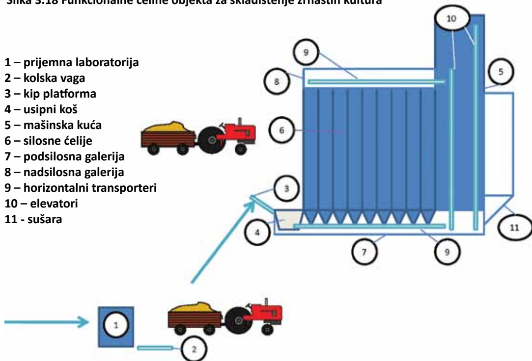
Slika 3.18 Funkcionalne celine objekta za skladištenje zrnastih kultura
