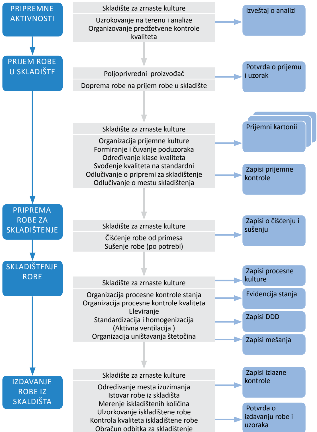
Slika 2.23 Dijagram toka tehnoloških procesa u skladištu za zrnaste kulture
