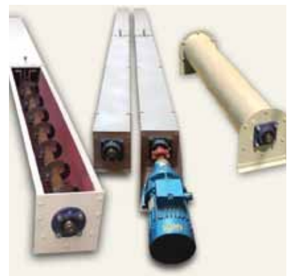
Slika 3.8 Izgled i šema pužnog transportera
