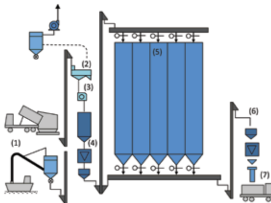
Slika 3.19 Funkcionalne celine objekta za skladištenje zrnastih kultura
