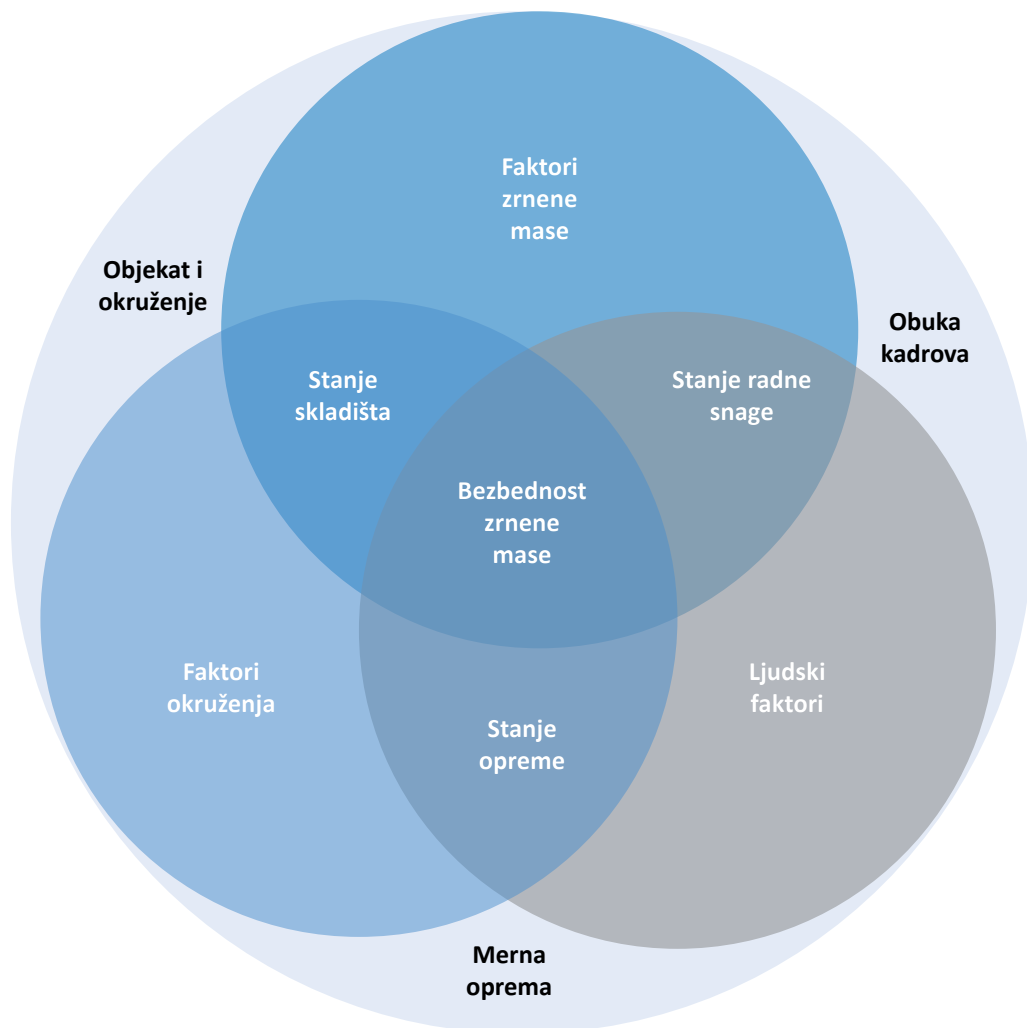
Slika 6.8 Shematski dijagram poljoprivredno–skladišnog ekosistema
