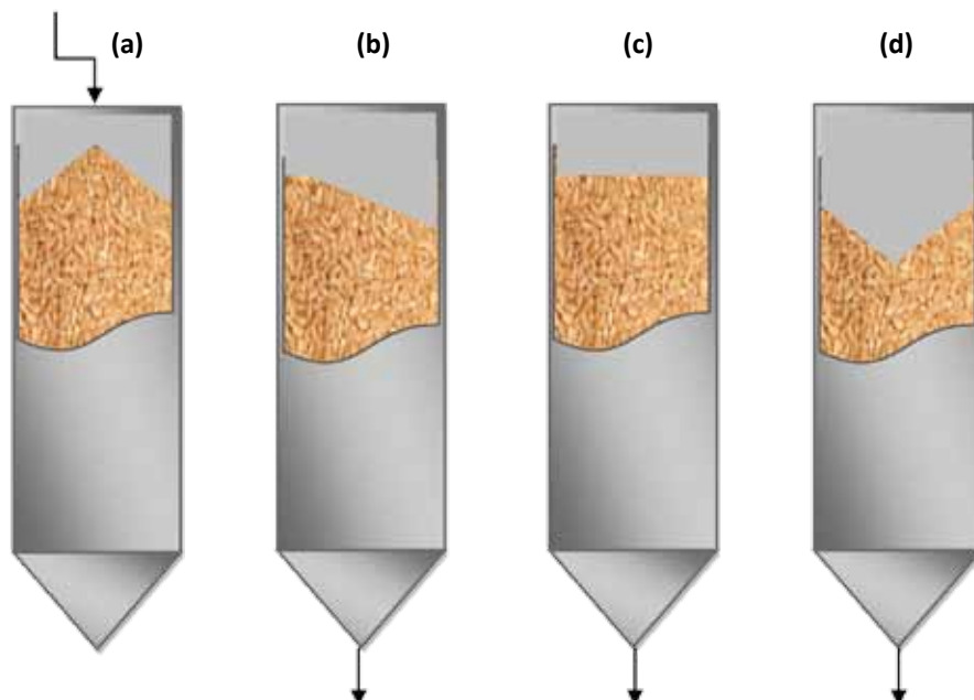
Slika 4.10 Mogući oblici gornje površine zrnene mase u ćeliji silosa
