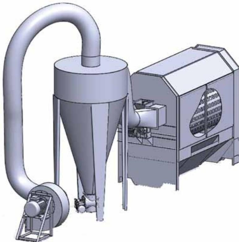
Slika 3.12 Šematski prikaz aspiracionog sistema
