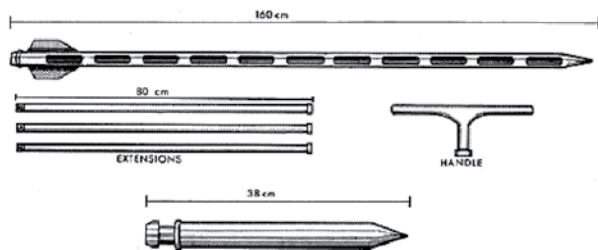
Slika 3.21 Sonde i šila za uzimanje uzoraka
