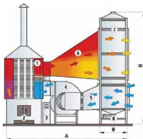
Slika 3.17 Presek sušare za zrno
