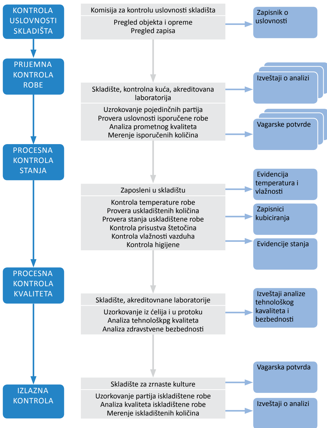
Slika 2.27 Dijagram toka procesa kontrole u skladištu za zrnaste kulture
