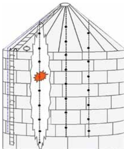
Slika 3.11 Presek uređaja za merenje temperature u ćelijama
