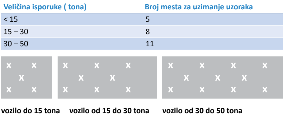
Slika 4.2 Broj i raspored mesta uzorkovanja zrnastih kultura iz transportnih sredstava
