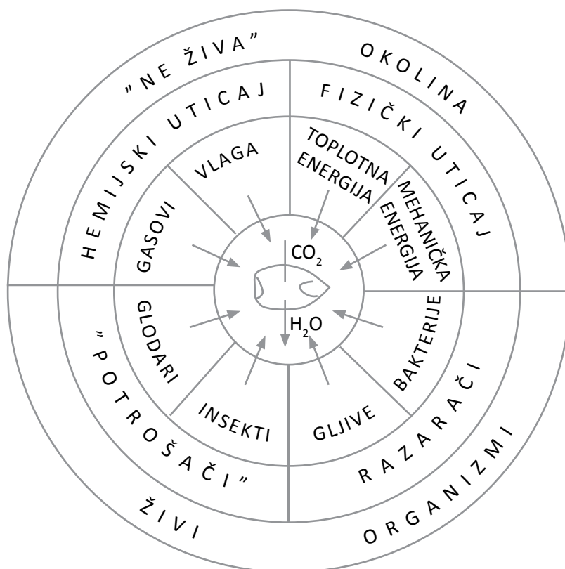
Slika 6.7 Šematski prikaz ekosistema uskladištenog zrna
