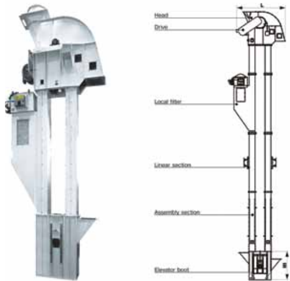
Slika 3.6 Izgled i šema elevatora
